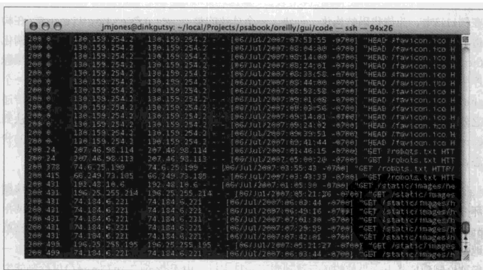
图11-3: Apache日志列表
